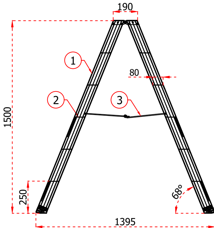
ESEVRPRO6 6 GRADINI
