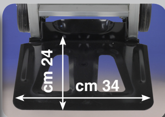
Pala ribaltabile in acciaio verniciato mm 240x340
