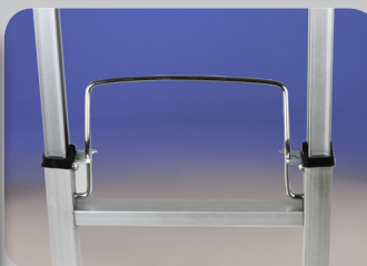
Meccanismo di chiusura del maniglione telescopico
