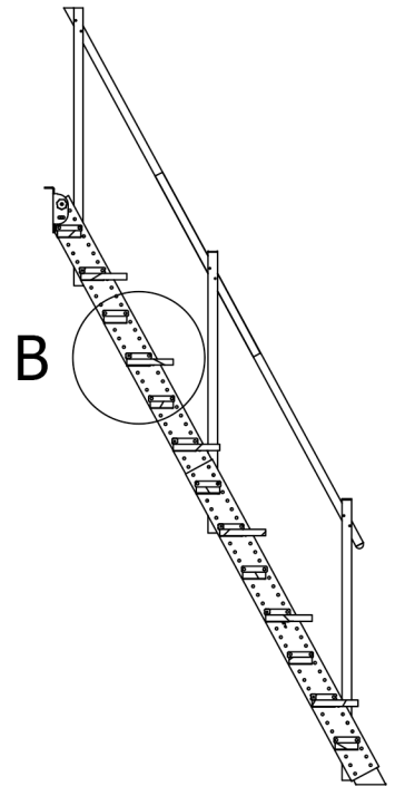
A-A ( 1 : 40 )
