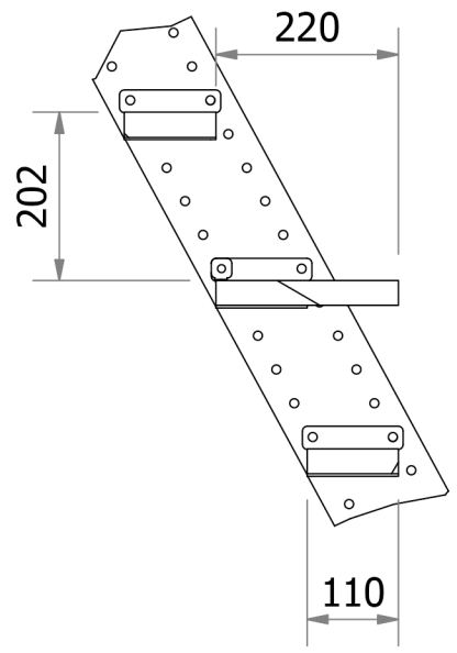
B ( 1 : 10 )
