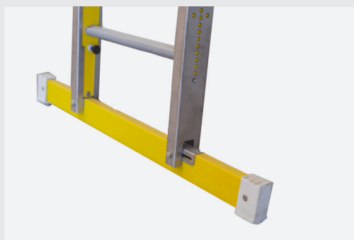
ESTABILIZADOR REGULABLE obligatorio para escaleras de más de 3 metros
