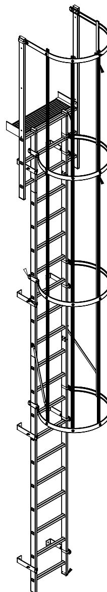
Escalera de 5,70 m. con peldaño de salida
