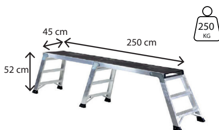
UPDOWNLM250: 50 cm x 45 cm x 52 cm
